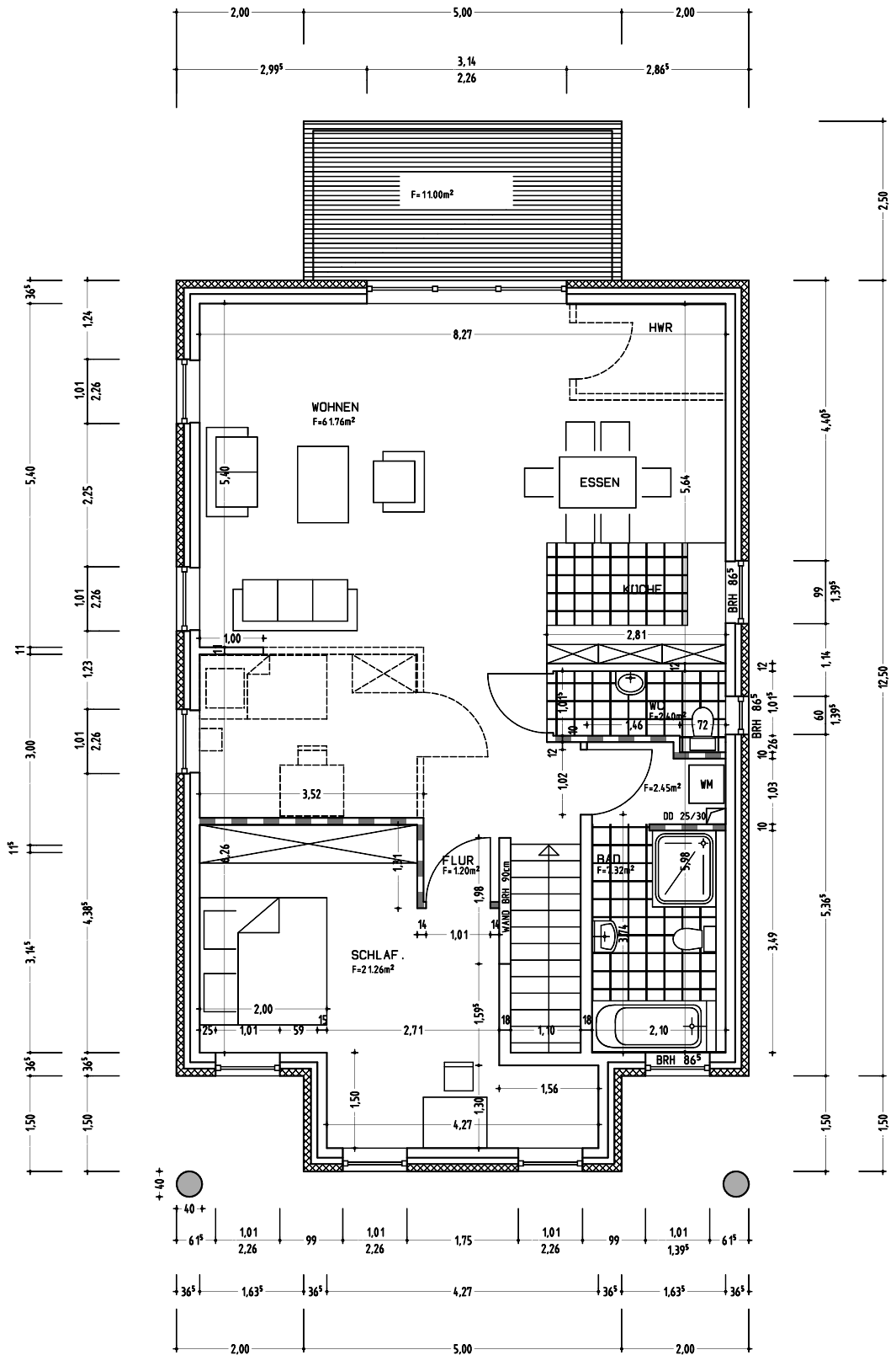
OBERGESHOSS HAUS 2
