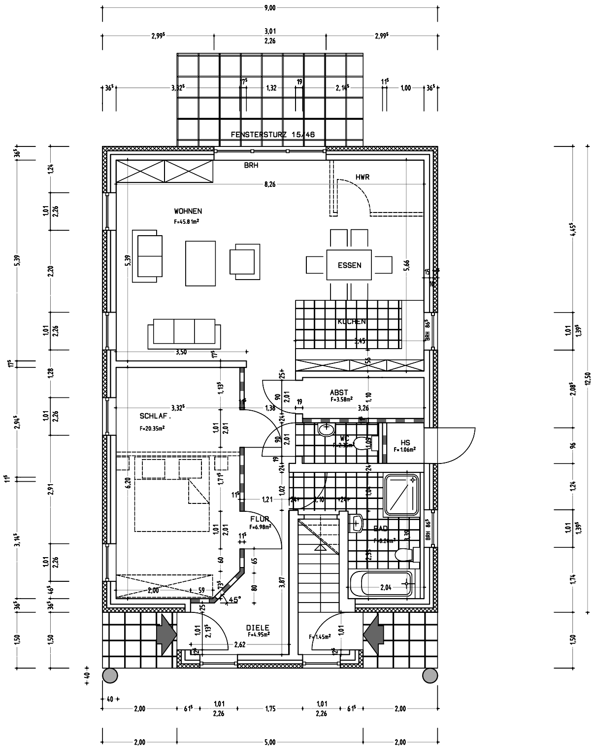
ERDGESHOSS HAUS 2
