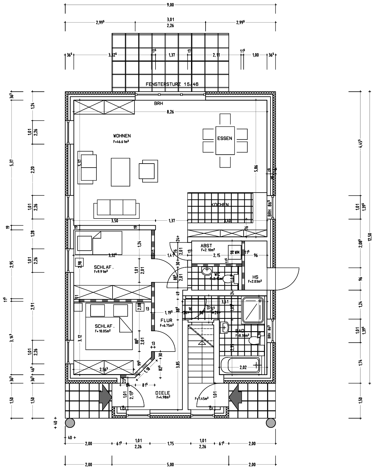
ERDGESHOSS HAUS 1
